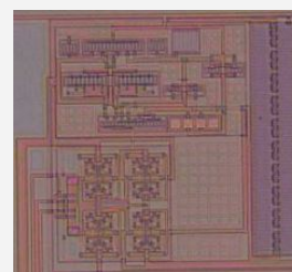
抵抗のばらつきが同相利得へ影響を与えない計装アンプのチップ写真
